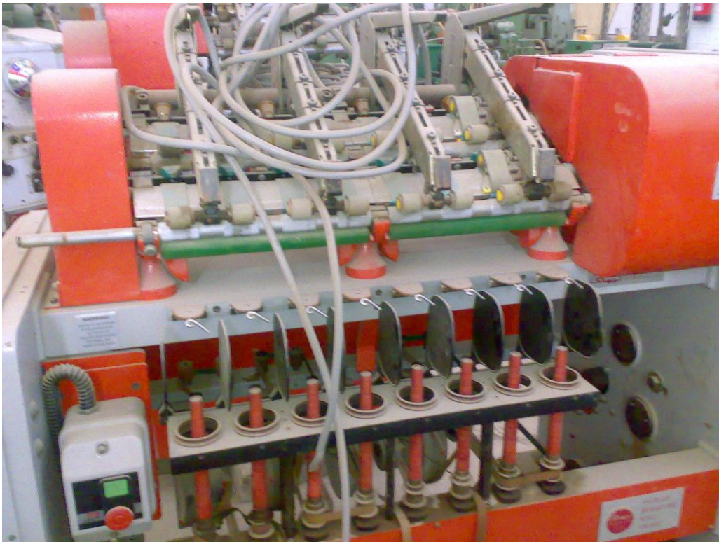
ماكينة الزوى Doubling / twisting machine
